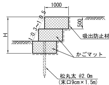
ふとん籠標準図
