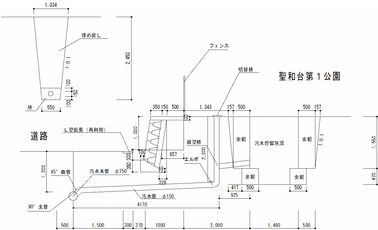
断面
