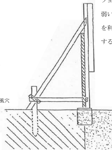
6 フェンス (a)
