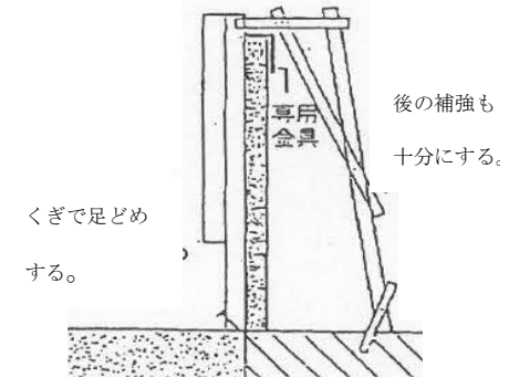
4 ブロック塀 (b)
