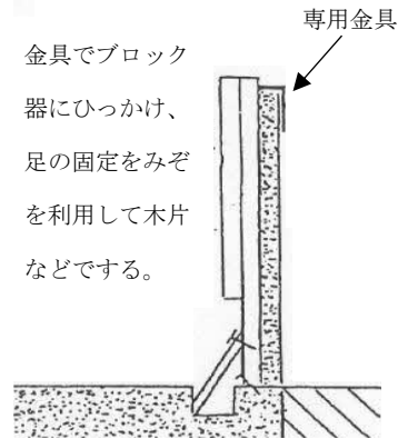
3 ブロック塀 (a)
