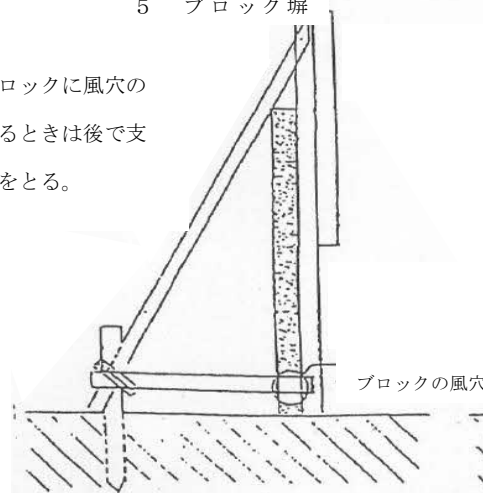
5 ブロック塀
