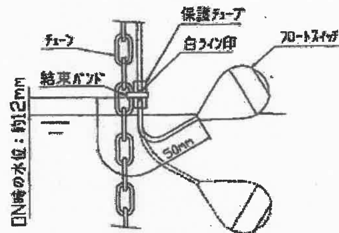
投入圧力式水位計
